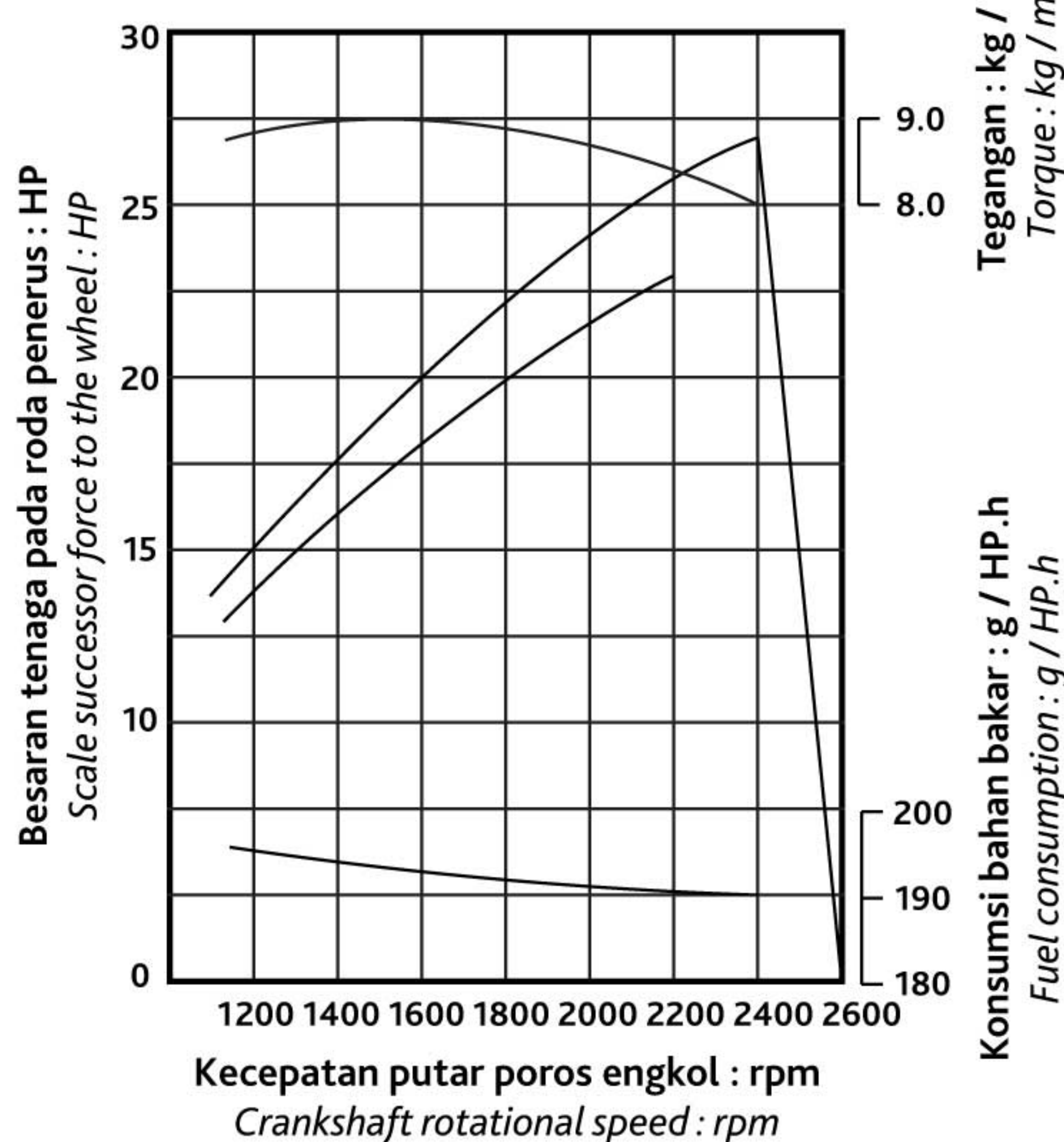
KURVA KINERJA DDI 2700 DDI 2700 PERFORMANCE CURVES
